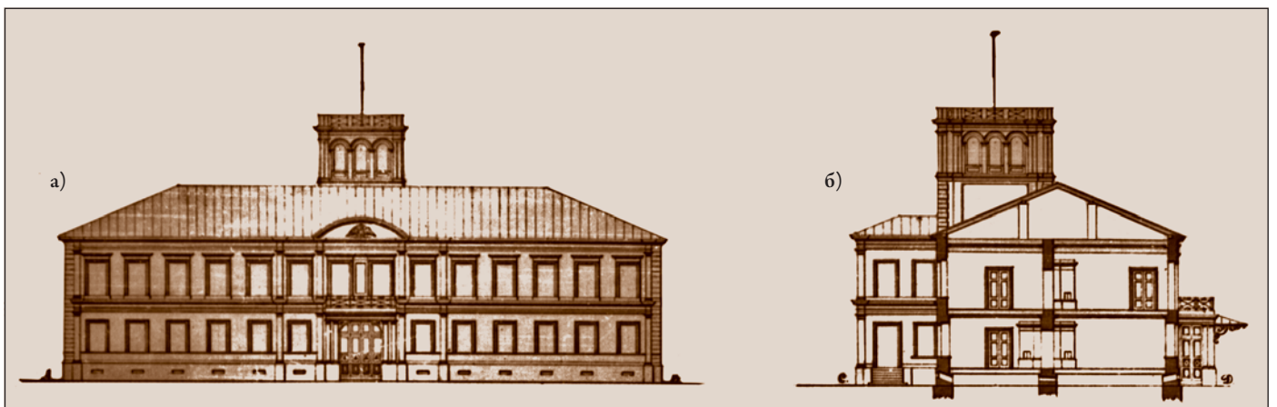
Генерал-губернаторский дворец: а) фасад, б) разрез. Из фондов РГИА.
